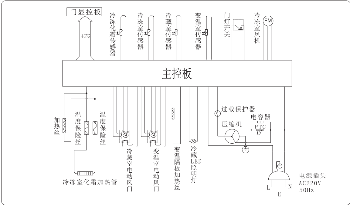
电路图(BCD-261WTEZW/BCD-263WTEW)
