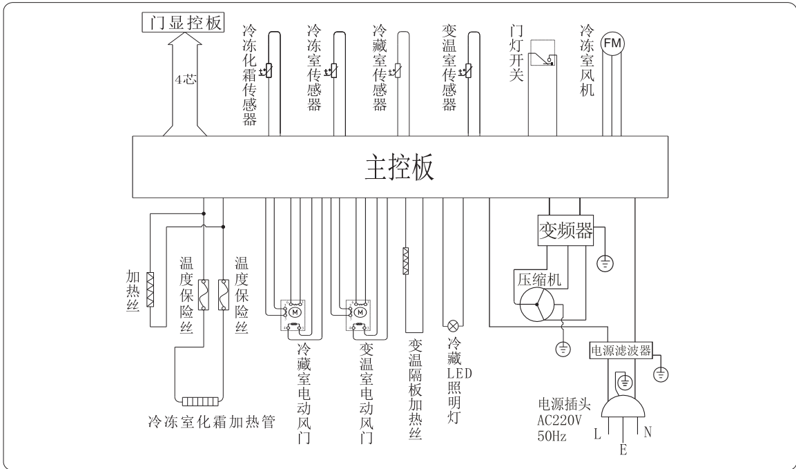
电路图(BCD-261WTBZW/BCD-263WTGBW)
